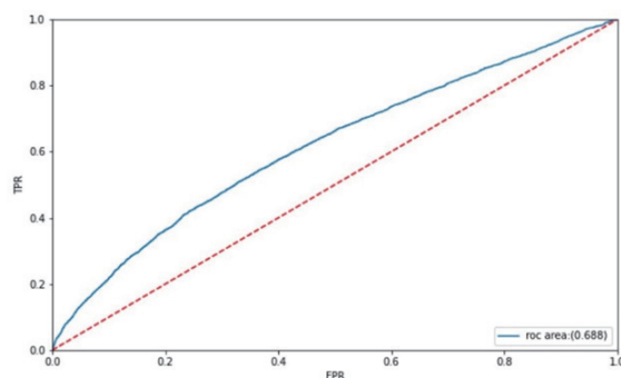
图 5 测试集 ROC 曲线
